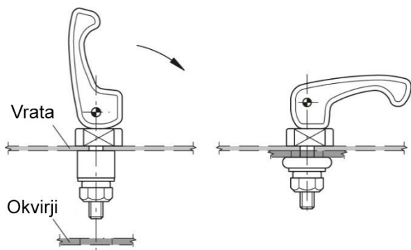
Vpenjanje elementov
